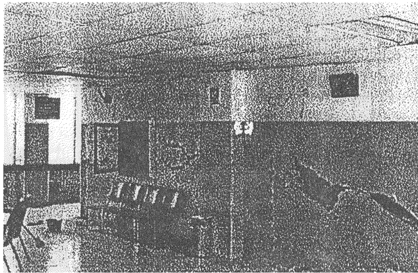
Foto 13. Agrietamiento en sala de espera junto a ascensores (Hosp. Miguel Alcivar)
