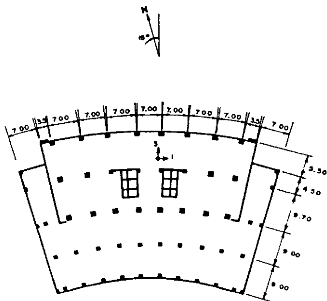
PLANTA SOTANO INSTITUTO COSTARRICENSE DE ELECTRICIDAD
