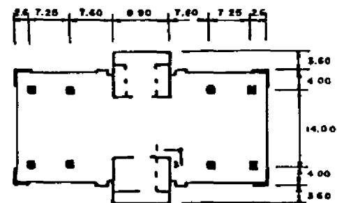
PLANTA PISO 17 BANCO NACIONAL DE COSTA RICA
