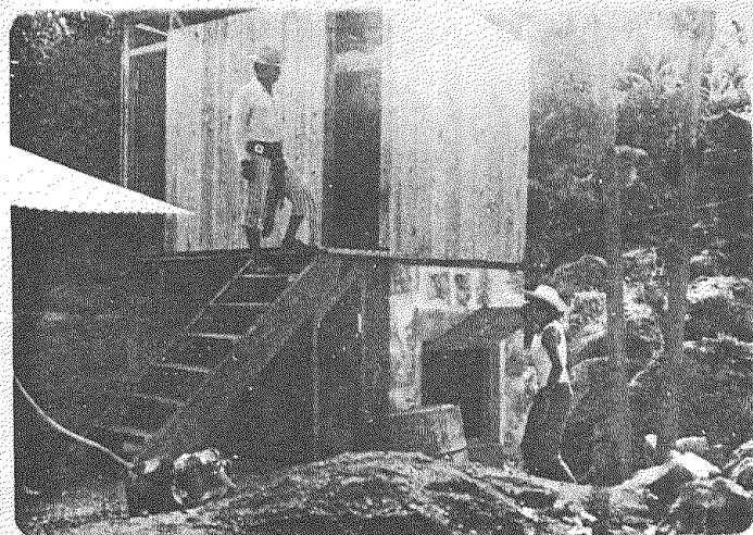
4.5 - LETRINA POR DESLIZAMIENTO
