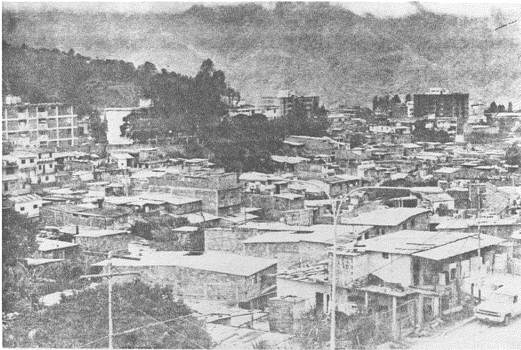
Foto 24.- Barrio Andrés Bello, constituido por viviendas aporticadas sin diseño sísmico de 1, 2 y 3 pisos localizado al borde de la Quebrada de los Chorros.
