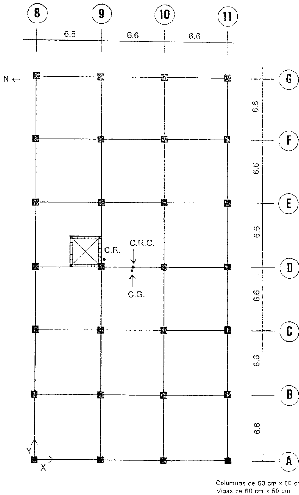
Figura A.7 HOSPITAL DE CURICO, CUERPO B - PLANTA PISOS 3, 4, 5. ESC. 1 : 250
