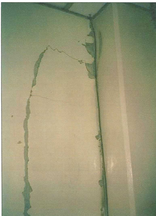
Foto 56: Daños en Encuentros de Muros con Pilar.
