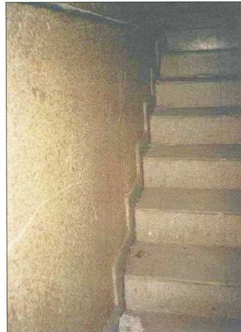
Foto 68: Daños en Muros de Caja Escala.
