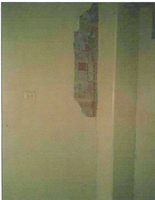
Foto 61: Daño Severo de Muro en Encuentro con Pilar.
