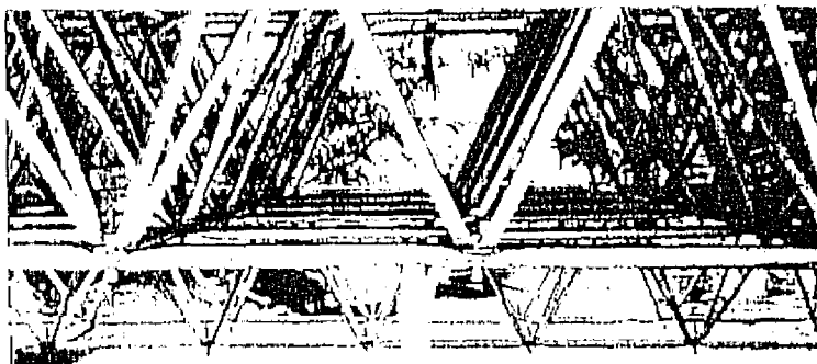
FOTO 30 Detalle del apoyo de la cubierta del área de emergencia.
