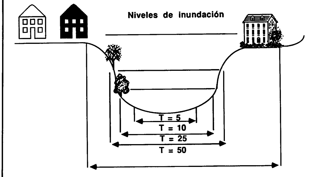
FIGURA 6 . CORTE TRANSVERSAL DE UN VALLE CON UNA PLANTA DE TRATAMIENTO.
